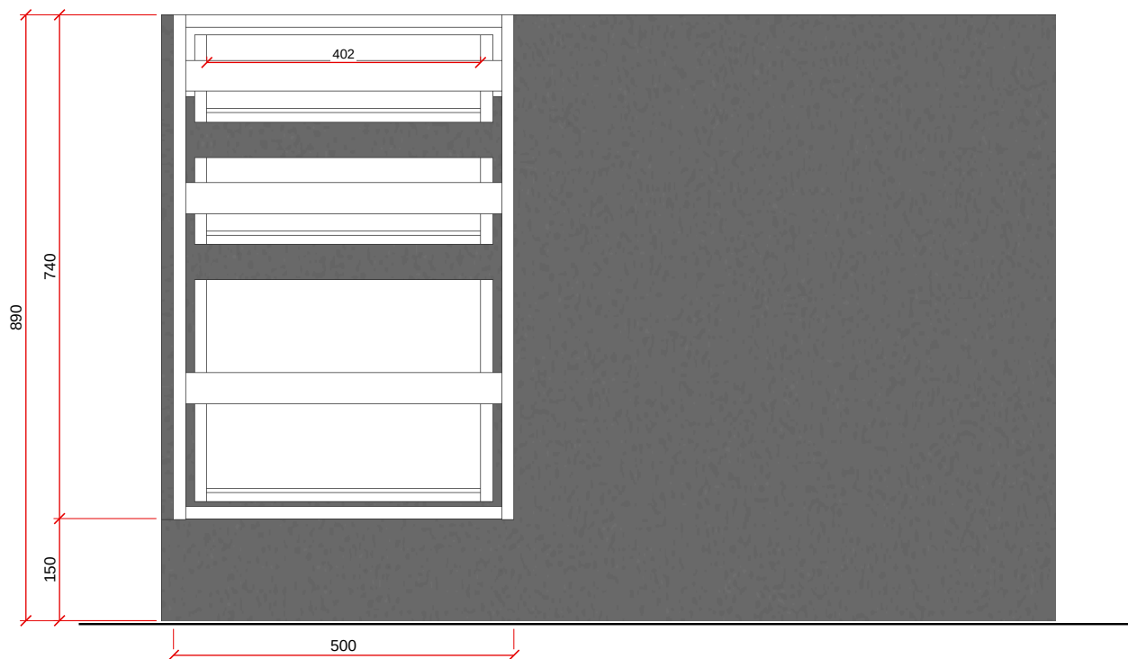
VISTA B - ESC. 1:10
